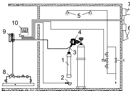
Рис. 1 Схема монтажа
